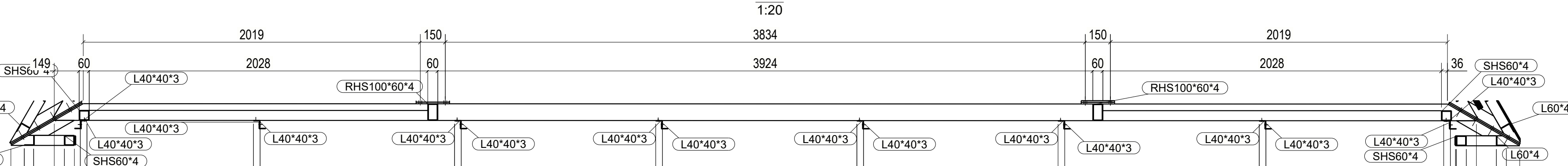
E - E 1:20
