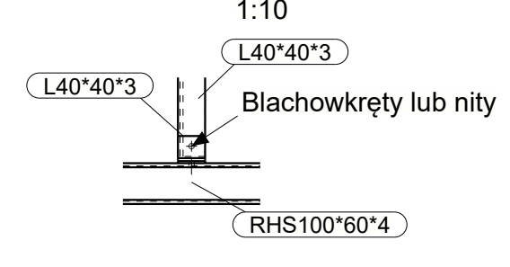
ŁĄCZENIE KATOWNIKÓW POD SIATKI 1:10
