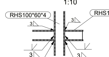
DETAL SPAWANIA RUR 1:10
