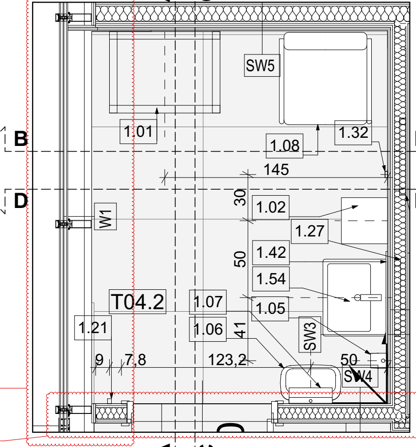
RZUT WĘZŁA SANITARNEGO T04- POSADZKI
