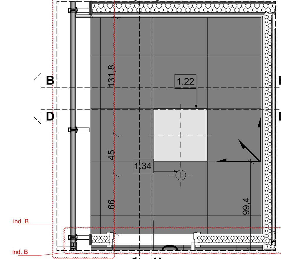
RZUT WĘZŁA SANITARNEGO T04- SUFIT
