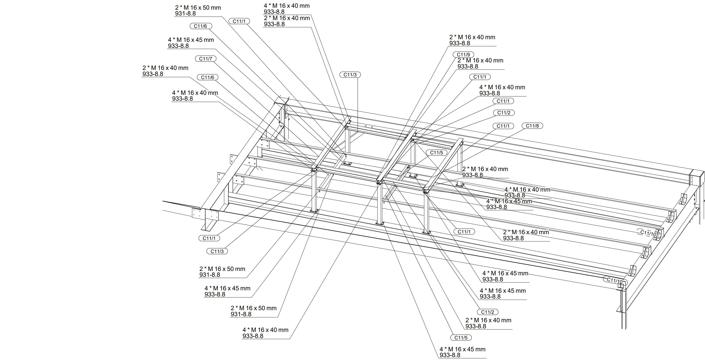
CENTRALA (OŚ 12-13/J-K) 1:50
