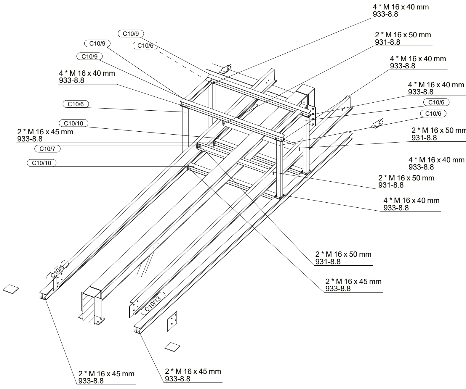
CENTRALA (OŚ 12-13/H-I) 1:50
