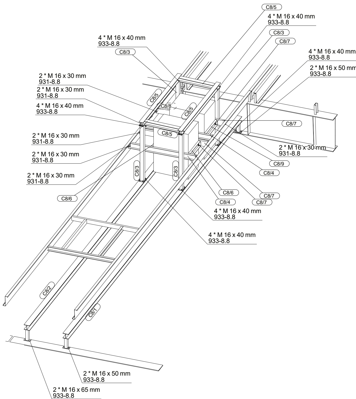
CENTRALA OŚ (12-13/B2-B3) 1:50
