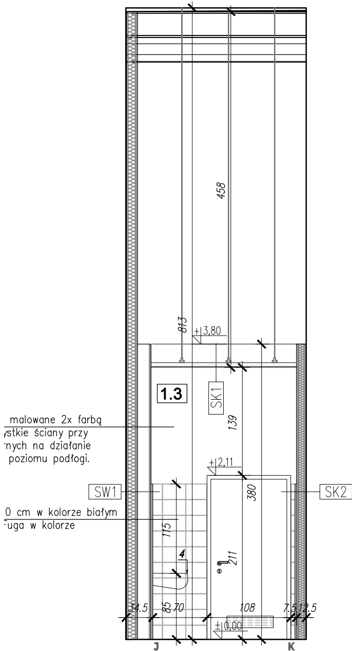
KŁAD ŚCIANY J-K
