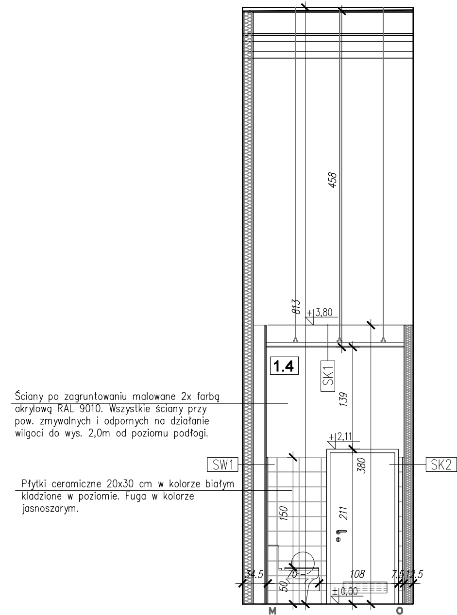
KŁAD ŚCIANY M-O
