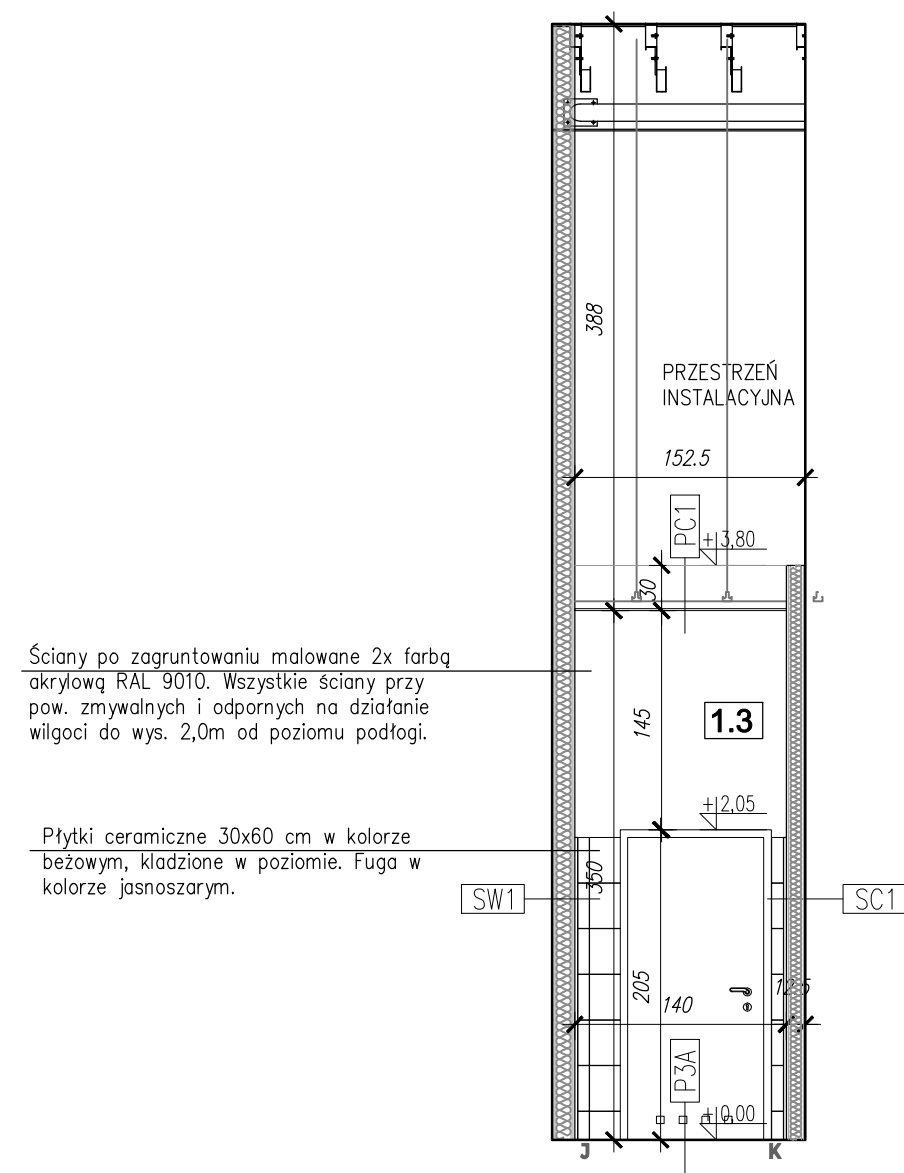
KŁAD ŚCIANY J-K
