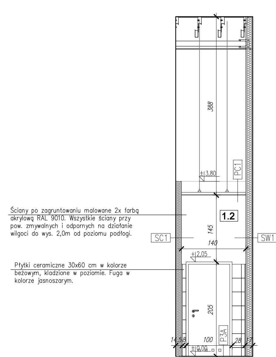
KŁAD ŚCIANY H-I
