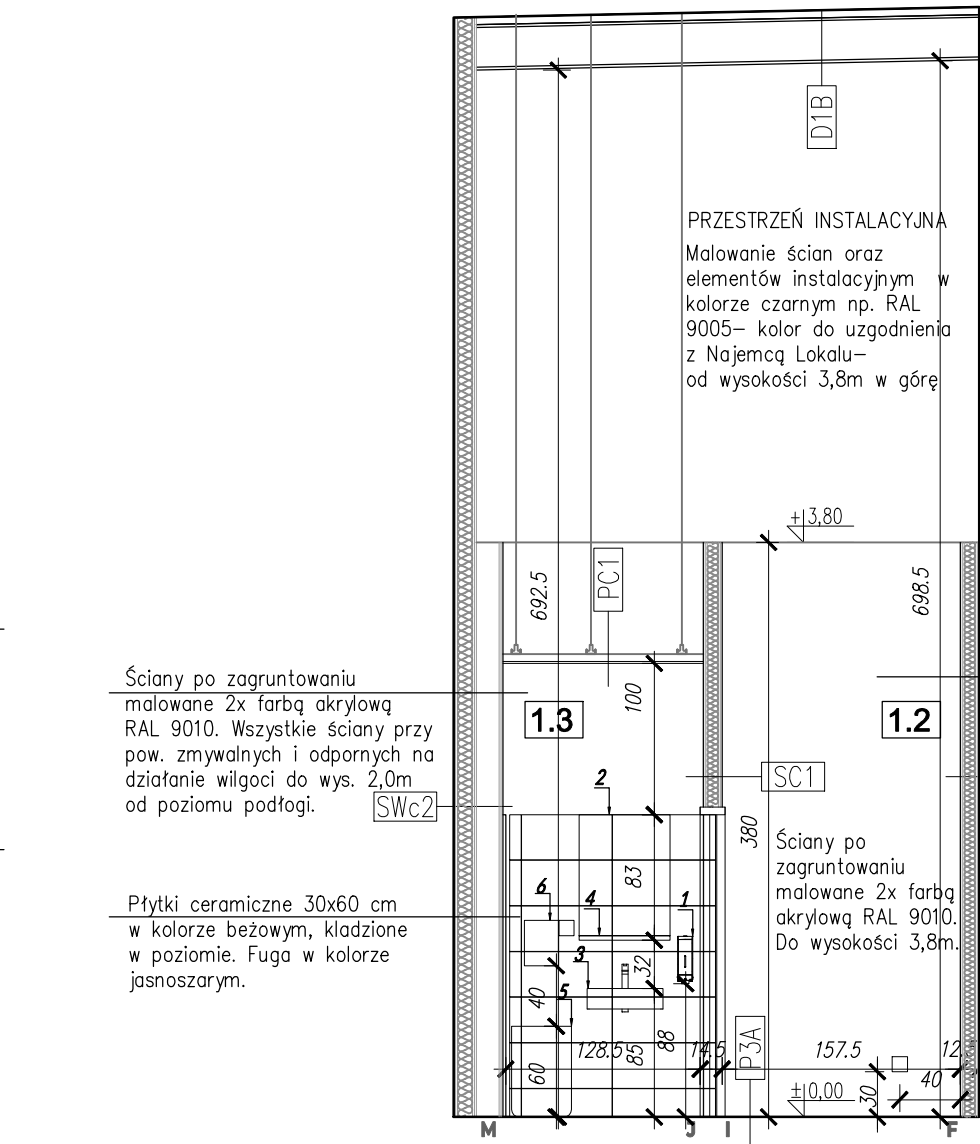
KŁAD ŚCIANY M-J, I-F
