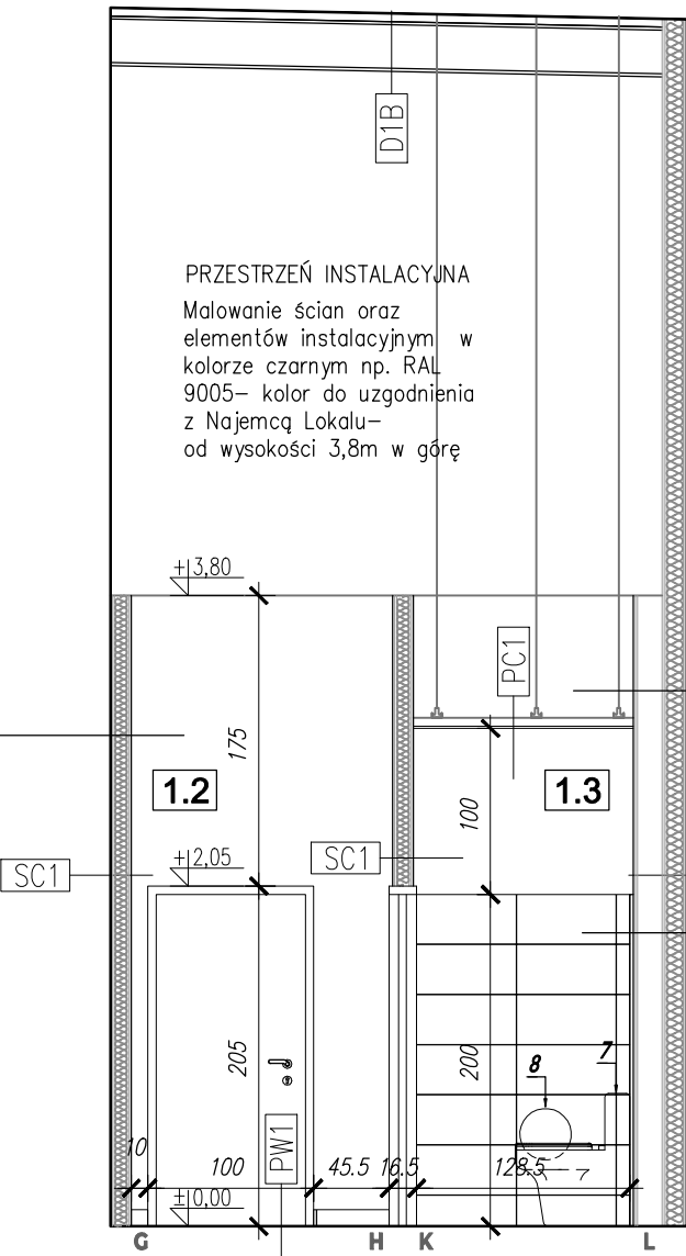
KŁAD ŚCIANY G-H, K-L
