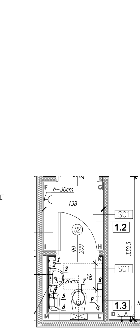
RZUT WC I ZAPLECZA
