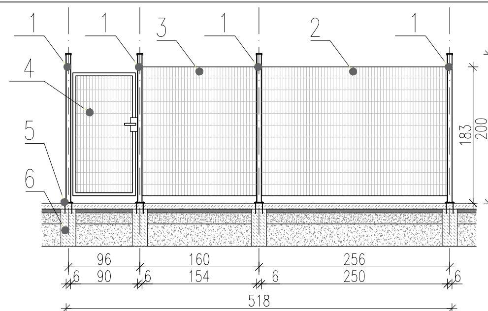
PRZEKRÓJ – SCHEMAT
