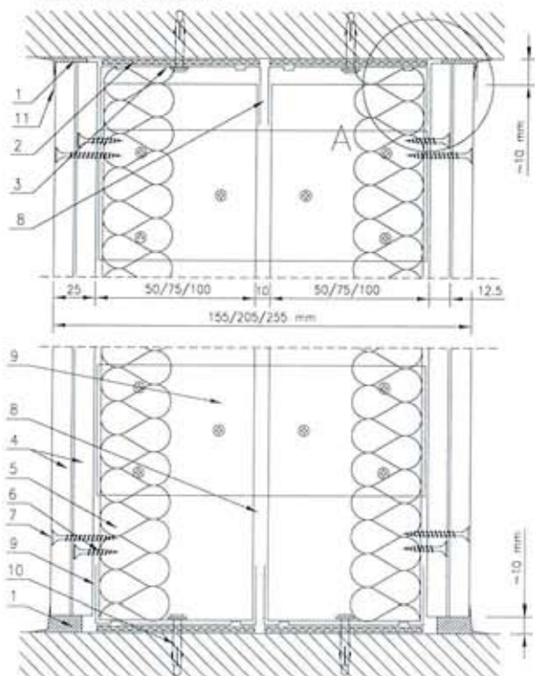
PRZEKRÓJ POZIOMY
