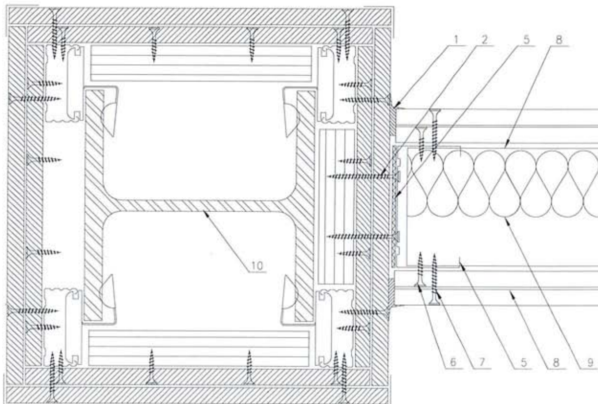
PRZEKRÓJ POZIOMY
