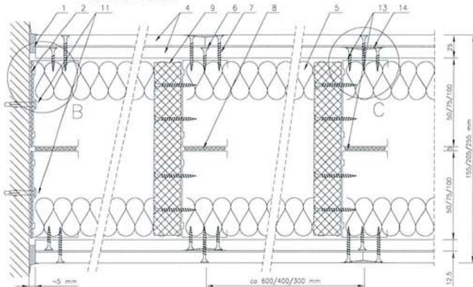
PRZEKRÓJ POZIOMY
