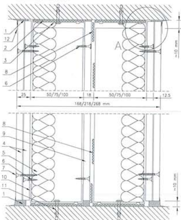
PRZĘKRÓJ POZIOMY
