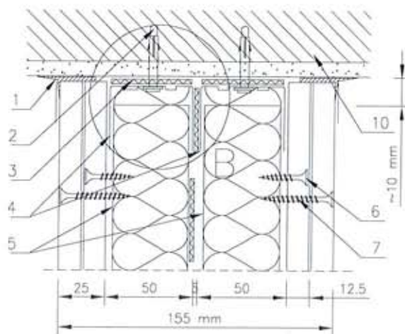
PRZEKRÓJ PIONOWY
