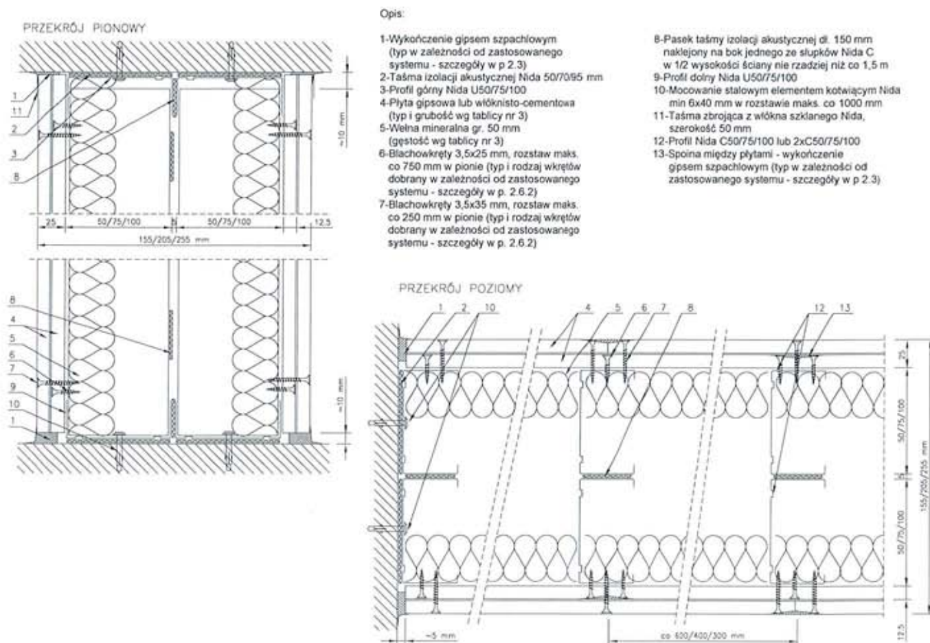
Rysunek Nr 3. Przekrój pionowy i poziomy ściany o podwójnej konstrukcji nośnej (rzędy profili przylegające) i podwójnym / potrójnym opływowaniu.
