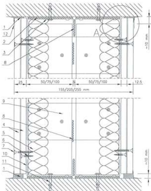
PRZEKRÓJ POZIOMY
