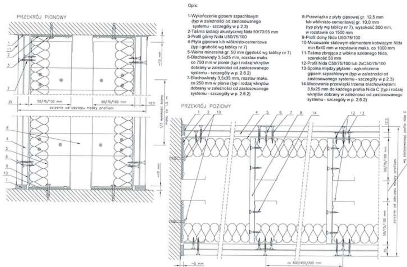
Rysunek Nr 7. Przekrój pionowy i poziomy ściany o podwójnej konstrukcji nośnej i podwójnym / potrójnym opływowaniu – instalacyjne.
