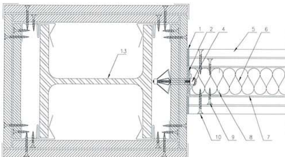
PRZĘKRÓJ POZIOMY
