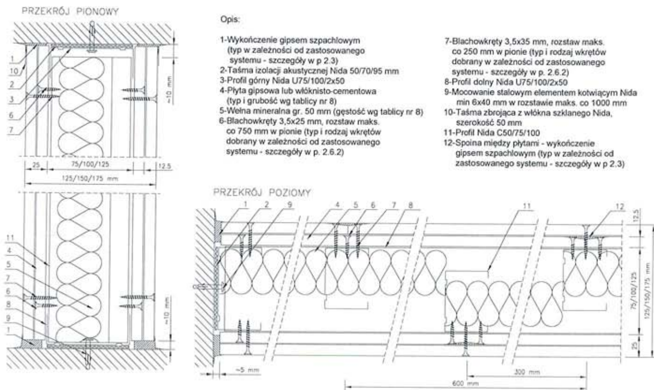
Rysunek Nr 8. Przekrój pionowy i poziomy ściany ze słupkami pojedynczymi rozmieszczonymi mijankowo i podwójnym / potrójnym opływowaniem.
