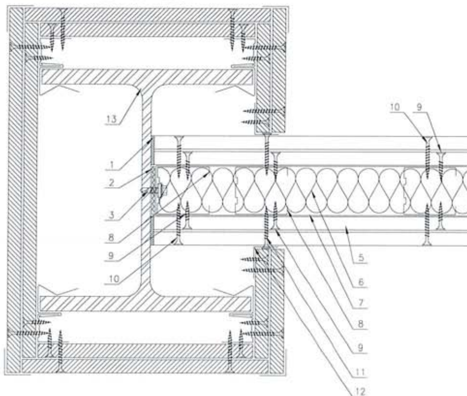
PRZĘKRÓJ POZIOMY
