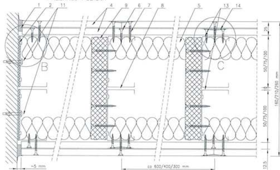
PRZEKRÓJ POZIOMY
