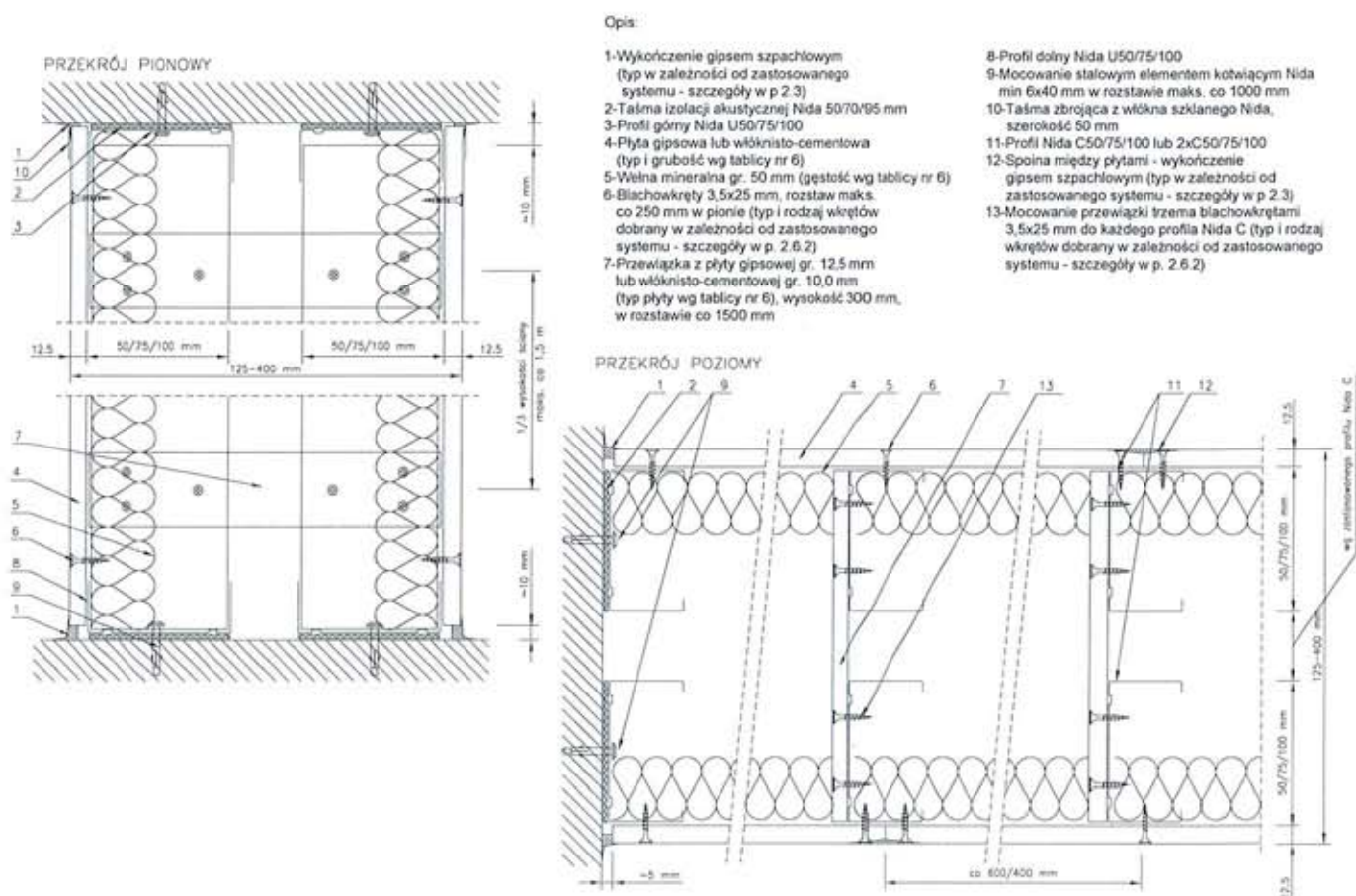
Rysunek Nr 6. Przekrój pionowy i poziomy ściany o podwójnej konstrukcji nośnej nośnej i pojedynczym oplytowaniu – instalacyjne.
