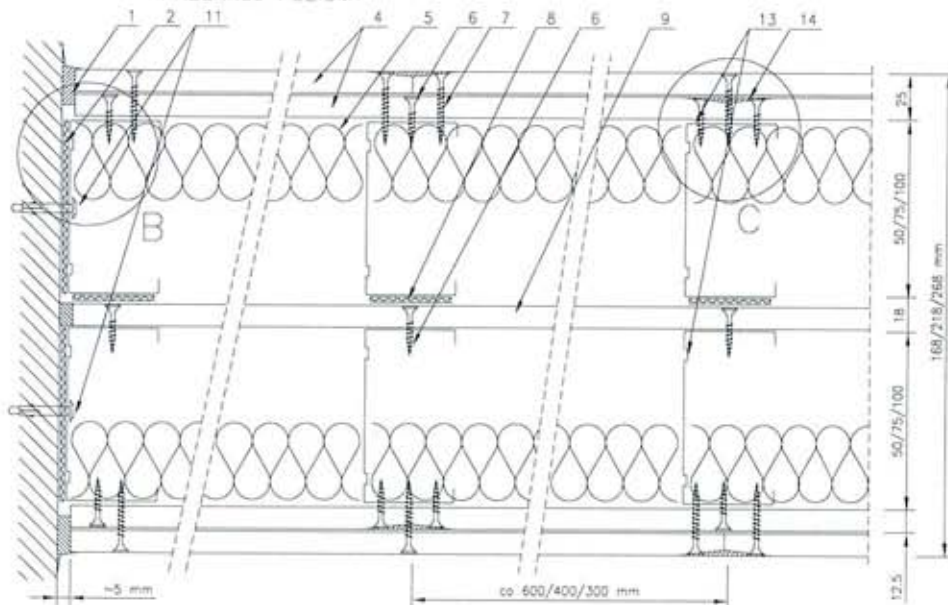
PRZĘKRÓJ POZIOMY
