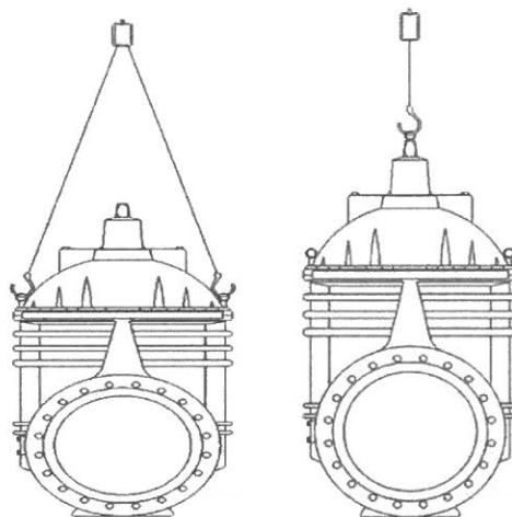
DN 500-600
