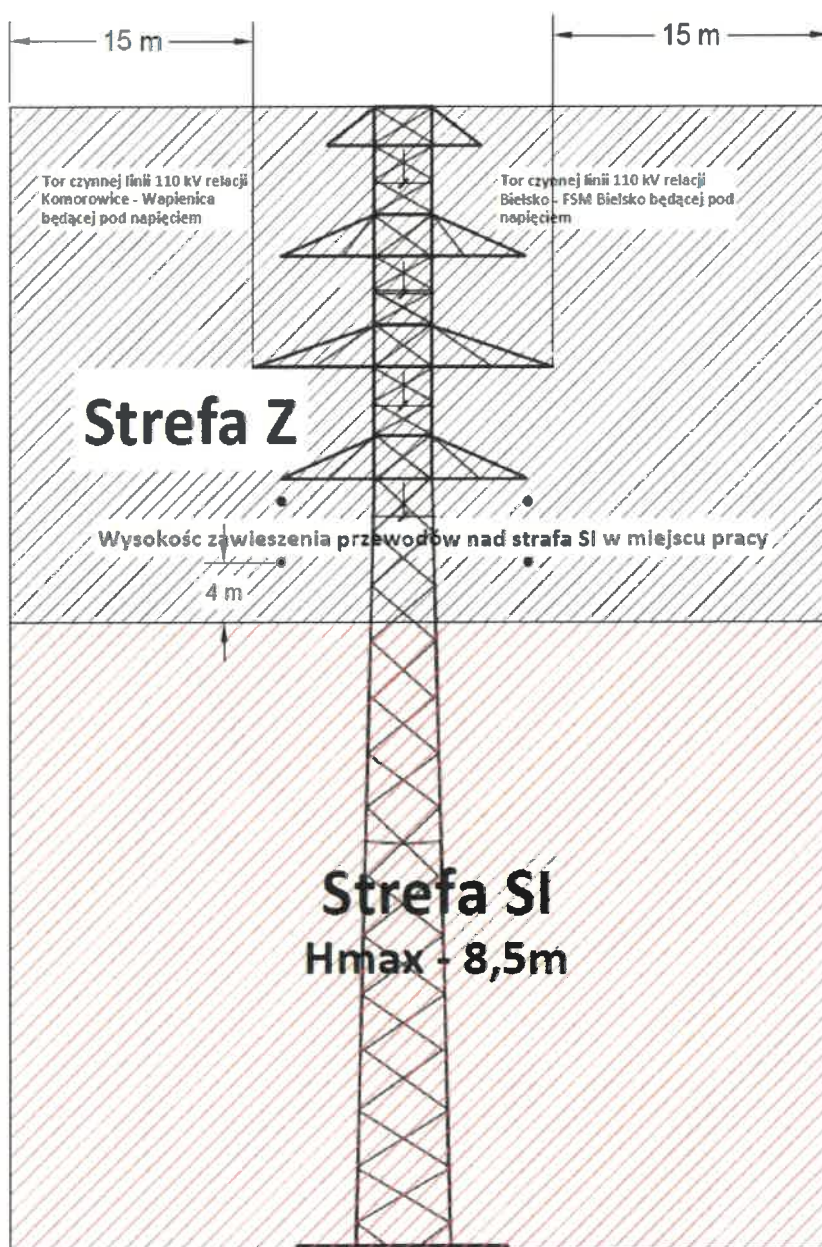
Rysunek 4—Podział stref wokół przewodów czynnych linii 110 kV (sylwetka słupa dwutorowego nr 17/2 linii Komorowice—Wapienica, Bielsko—FSM Bielsko— Tor lewy orientacja w stronę słupa 17/1 linia Komorowice—Wapienica, Tor prawy orientacja w stronę słupa 17/1 linia Bielsko—FSM Bielsko)
