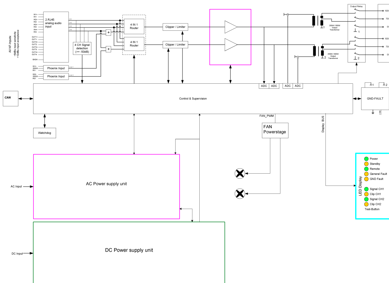
Rys. 1: Schemat elektryczny
