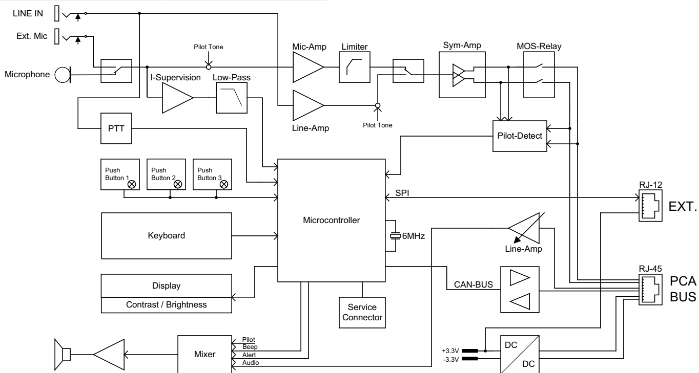
Rys. 1: Schemat elektryczny
