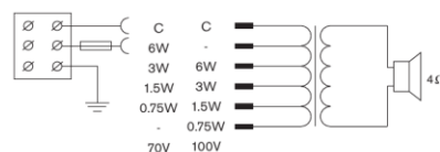
Schemat połączeń
