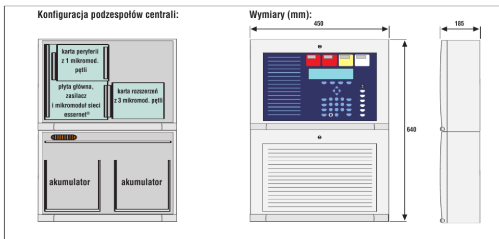
Konfiguracja podzespołów centrali i wymiary
